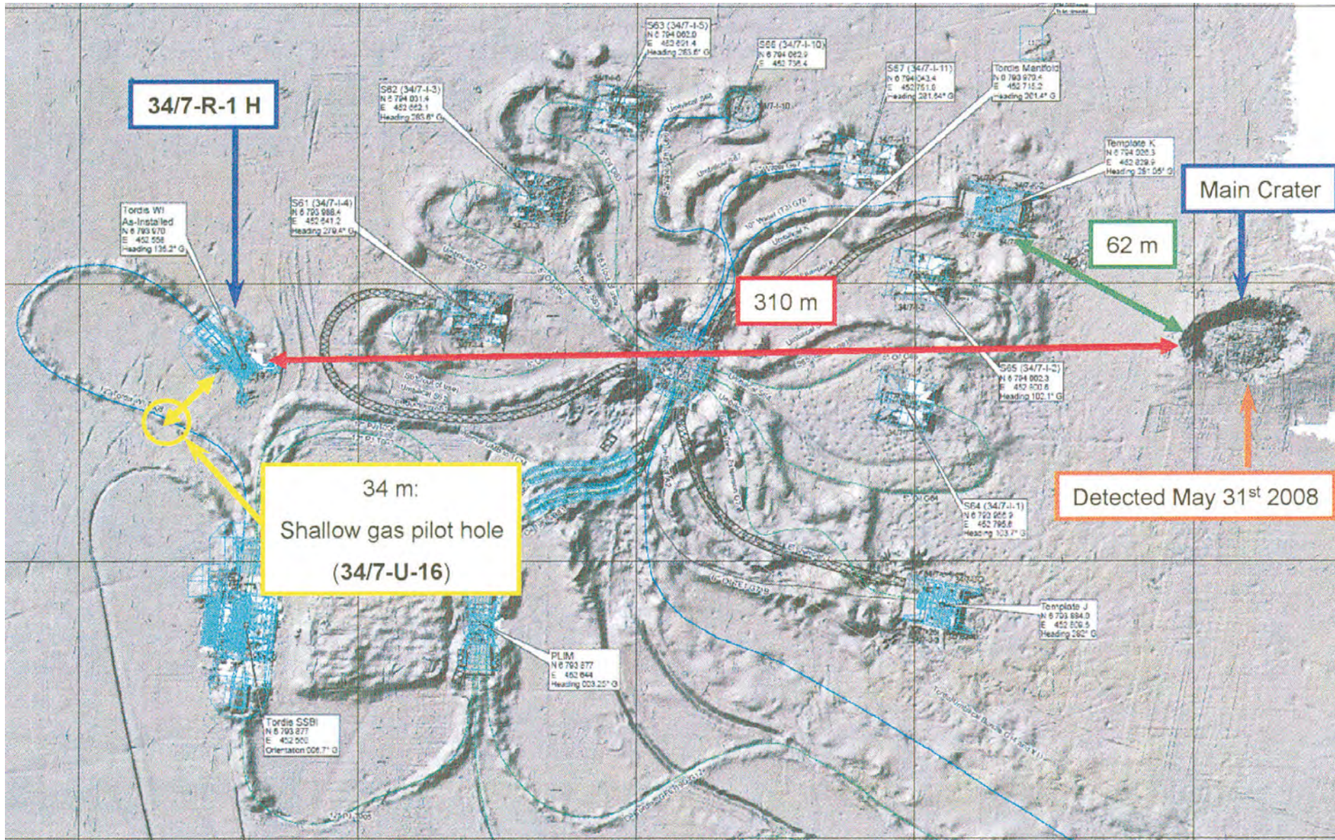
Fig. 1 Tordisfeltet med havbunnsinnretninger og rørledninger. Gropen på havbunnen er helt til høyre i bildet (62 m fra nærmeste bunnramme). Kilde: Statoil
