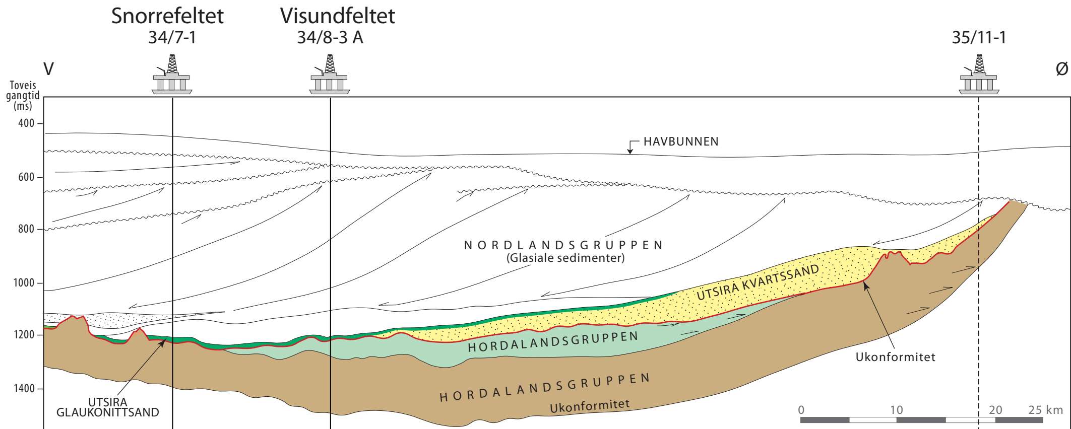
Fig. 4: Øst-vest seismisk profil over Tampen-området i nordlige Nordsjøen som blant annet viser tykkelsen av Utsiraformasjonen på Snorre- og Visundfeltet. Profilets beliggenhet er vist på Fig. 3.
