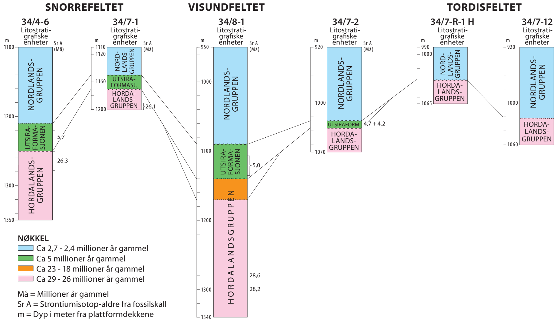
Fig. 5: Korrelasjon av lithostratigrafiske enheter mellom brønnene 34/4-6 (Snorrefeltet), 34/7-1 (Snorrefeltet), 34/8-1 (Visundfeltet), 34/7-2, 34/7-R-1 H (Tordisfeltet) og 34/7-12 (Tordisfeltområdet) på Tampenområdet i nordlige Nordsjøen. Figuren viser at Utsiraformasjonen blir mye tynnere i retning sydover fra Snorrefeltet (34/4-6, 34/7-1) og Visundfeltet (34/8-1) mot Tordisfeltområdet (34/7-2) og mangler helt på selve Tordisfeltet (34/7-R-1 H, 34/7-12)
